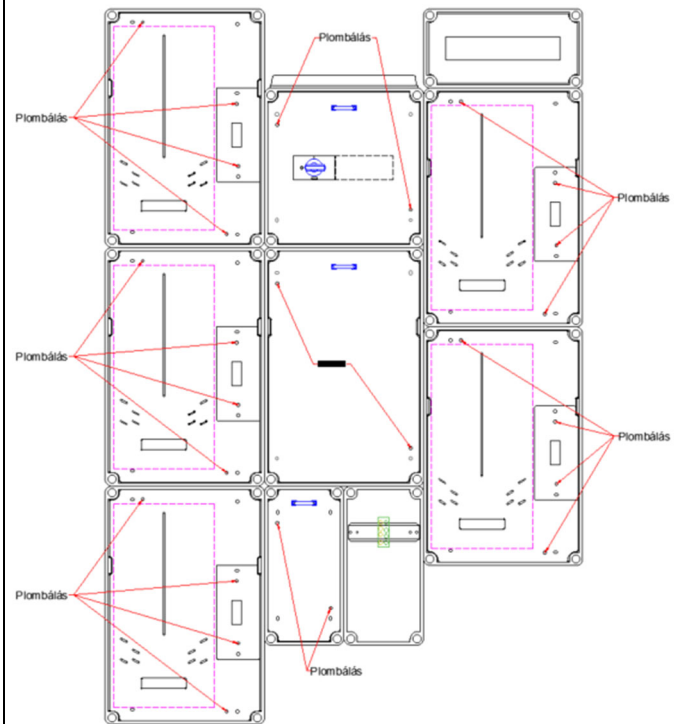
ELRENDEZÉSI RAJZ PLOMBÁLÁSI HELYEKKEL (kizárólag jó minőségű):
